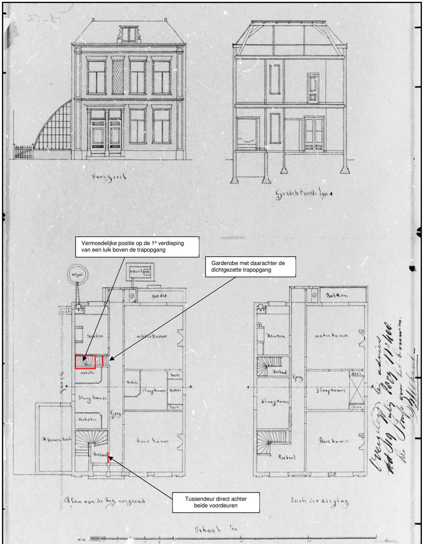
Detail Bouwplan van Maliebaan 72, tekening uit 1879, Bron: Utrechts Archief; 1879.0722b. Li-boven, tegen de klok in: Voorgevel, Begane grond, Verdieping (beiden met doorsnede-stippellijn A-A, en Doorsnede naar achteren. Typisch dat er een tussendeur was achter de voordeuren en 2 trappen van BG naar 1 e verdieping. Voor dubbele bewoning? In de doorsnede (boven rechts) is duidelijk de verdiepte aanleg van het linker woningdeel t.b.v. de kelder te zien, In rood zijn door GJvW een aantal latere aanpassingen ingetekend.
